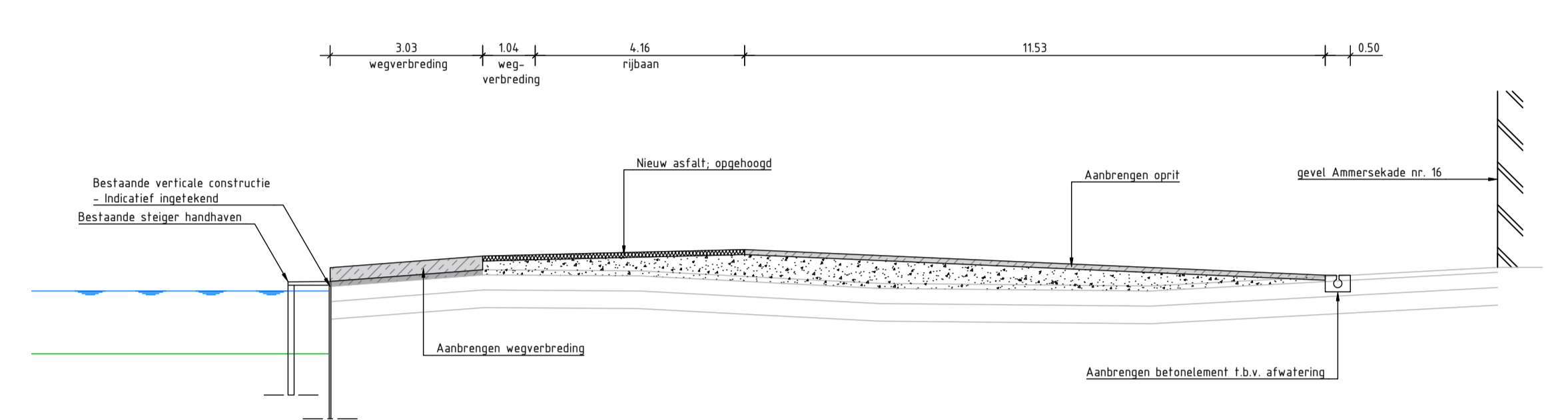
DWARSPROFIEL 9 (variant 1) schaal 1:100
