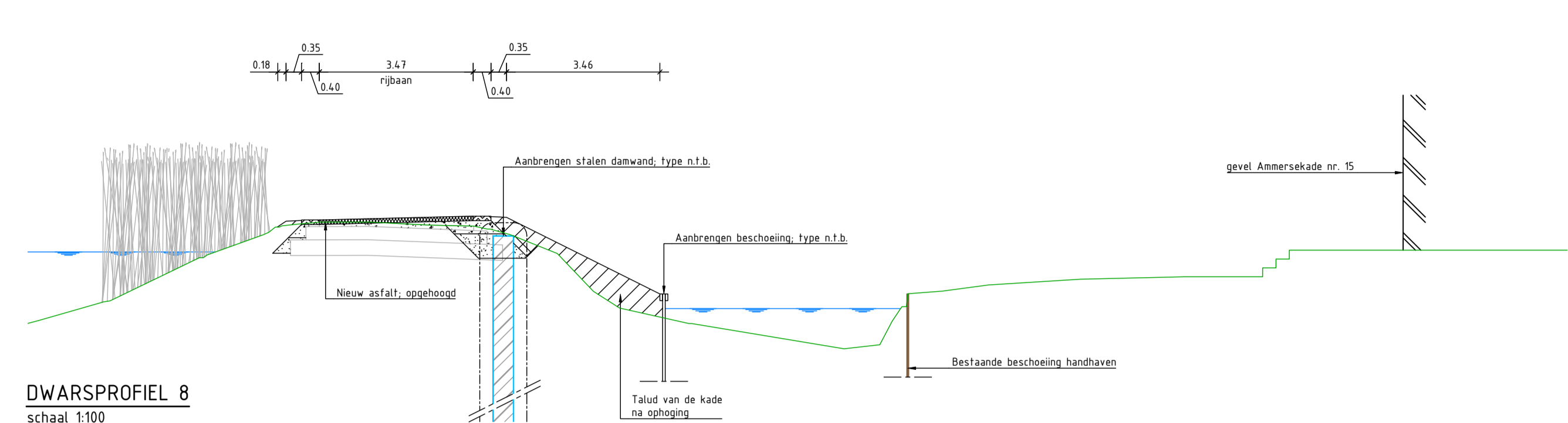
DWARSPROFIEL 8 schaal 1:100
