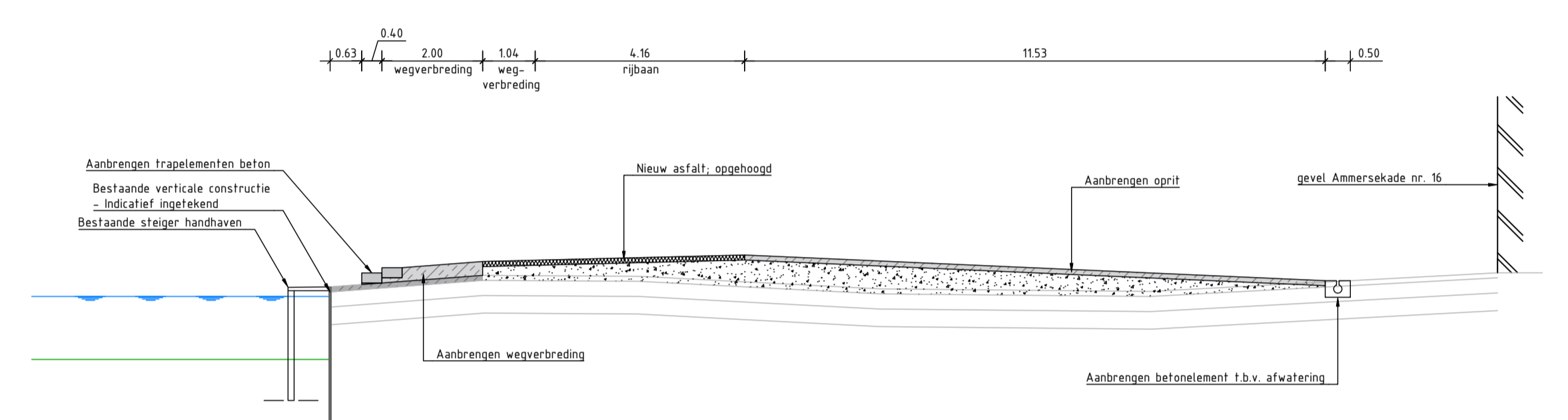
DWARSPROFIEL 9 (variant 2) schaal 1:100
