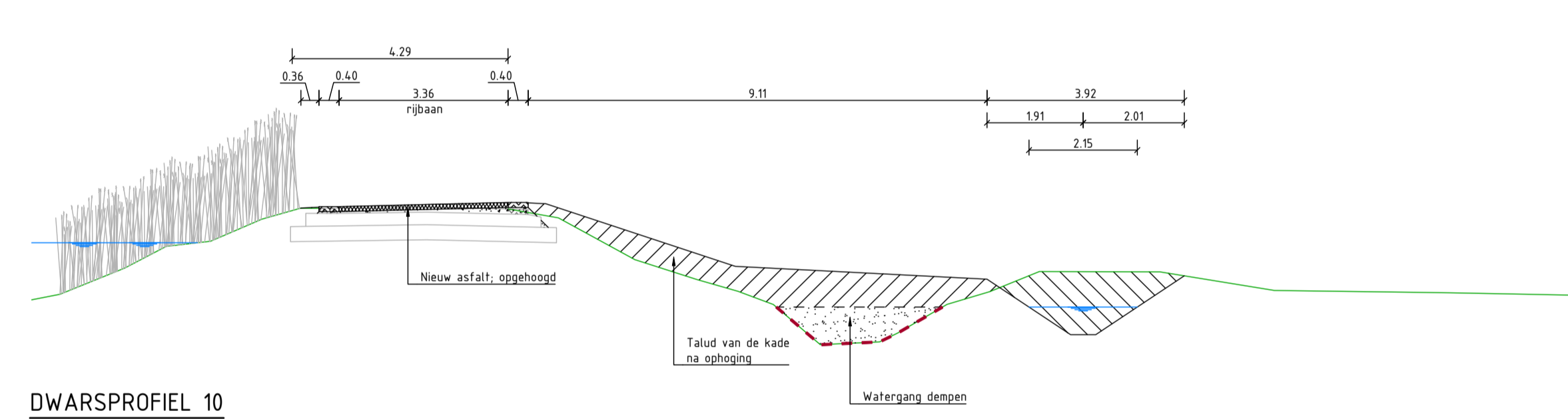
DWARSPROFIEL 10 schaal 1:100
